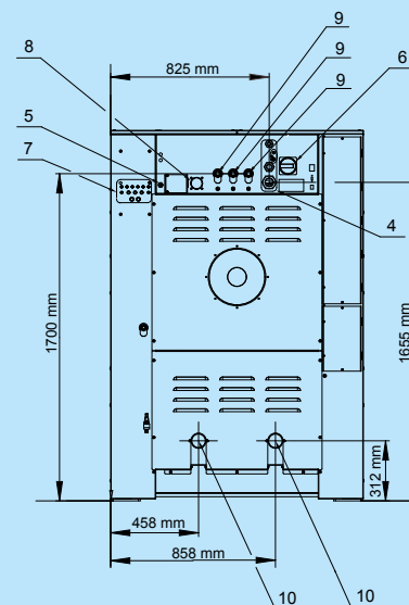
Задняя панель
