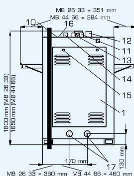
ВИД СЗАДИ MB 66
