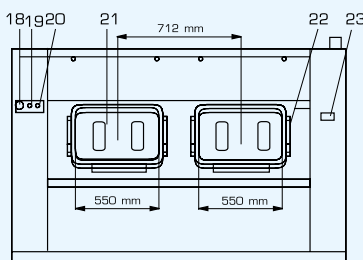
ВИД СЗАДИ MB 66
