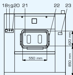
ВИД СЗАДИ MB 26 33 44
