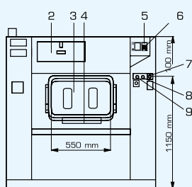
ВИД СПЕРЕДИ MB 26 33 44
