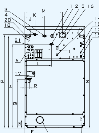
Вид сзади
