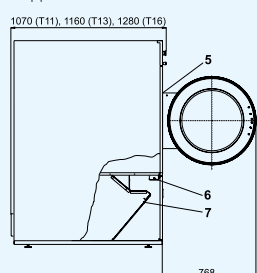
ВИД СБОКУ Т 11 13 16
